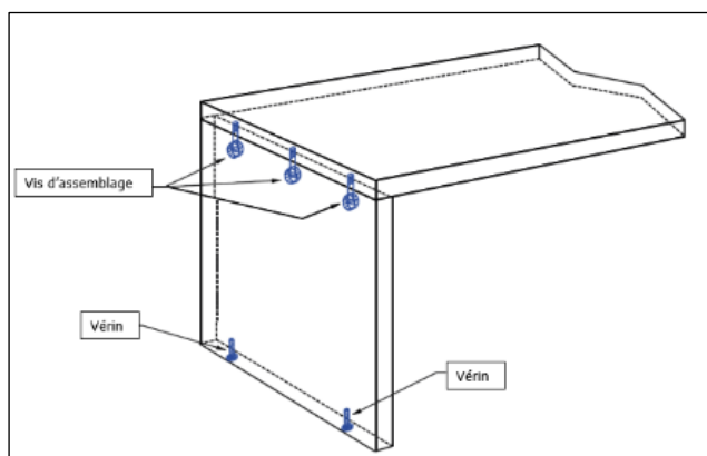
Système de fixation jambage simple
